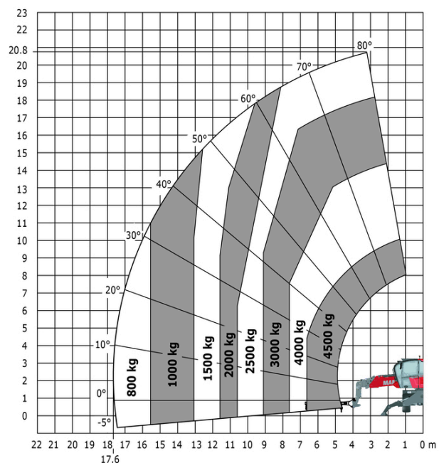
Macchina su stabilizzatori abbassati con gancio 5000 kg (metrico)
