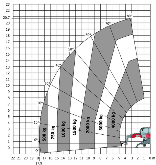
Macchina su stabilizzatori abbassati con braccio da 4000 kg (sistema metrico)
